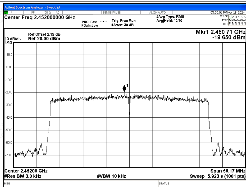
PSD NVNT ax40 2452MHz Ant6
