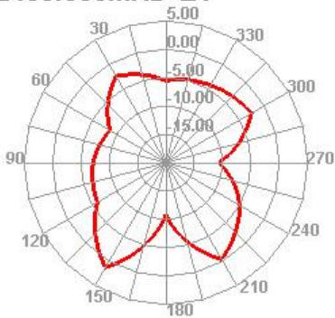
2450.000MHz
