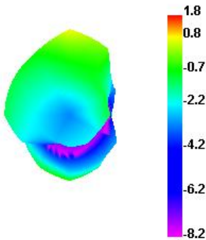
2400.000MHz E1
