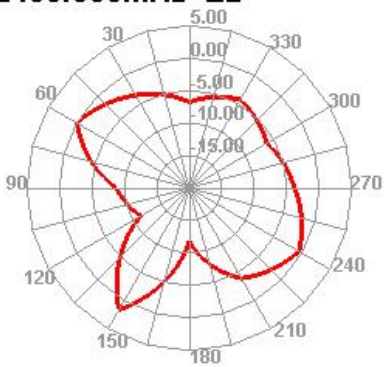
2450.000MHz E2
