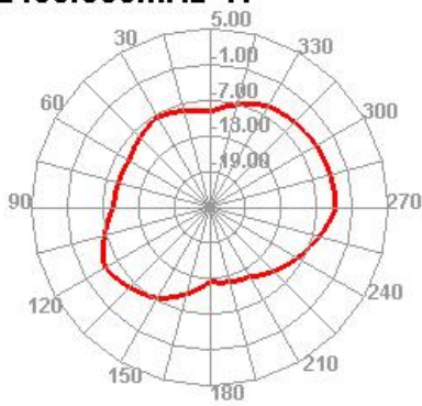
2450.000MHz H
