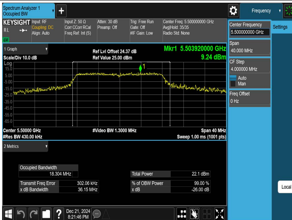
11A-Ant1-5500
