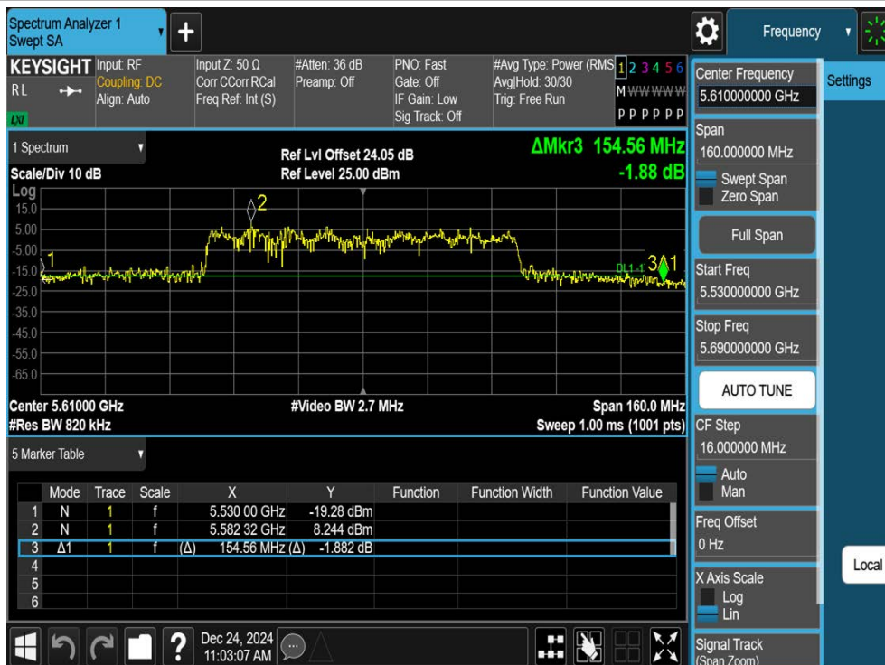
11AC80SISO-Ant1-5610
