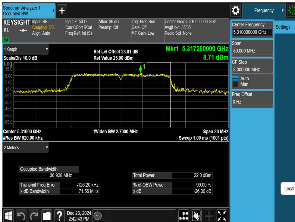
11N40SISO-Ant1-5310
