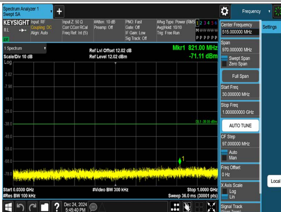
11G-Ant1-2437-30~1000-PASS
