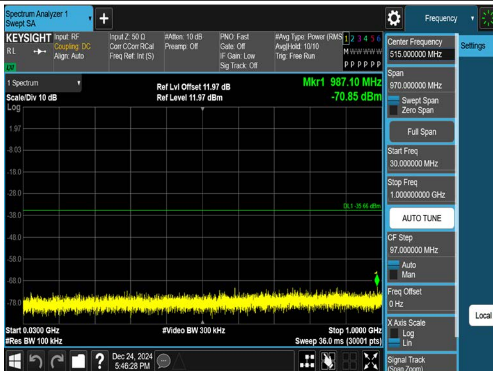
11G-Ant1-2462-30~1000-PASS
