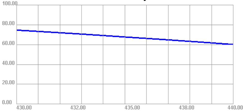
430.00MHz - 440.00MHz Efficiency
