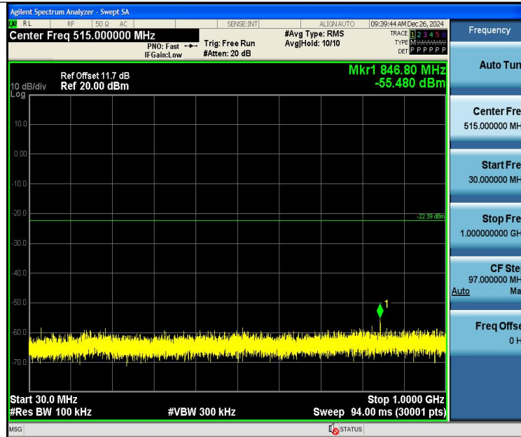
BLE_2M-Ant1-2480-30~1000-PASS
