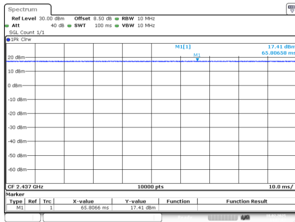
802.11b_2437MHz_Chain 0
