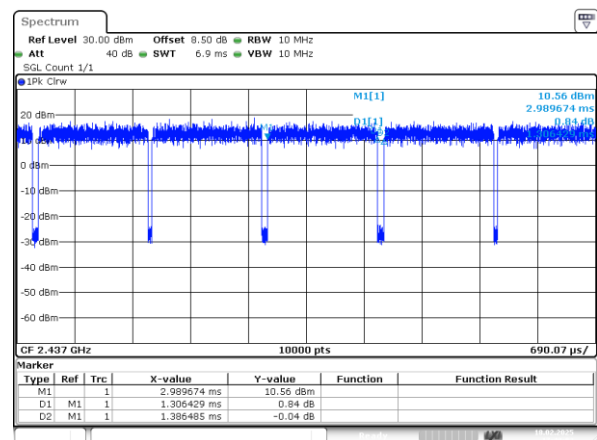
802.11n20_2437MHz_Chain 1
