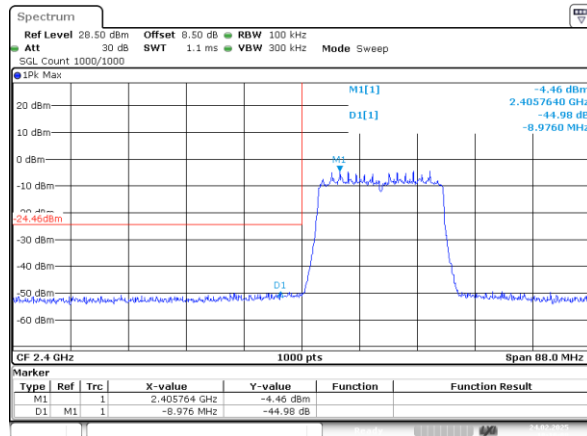
802.11ax20_2412MHz_Chain 1
