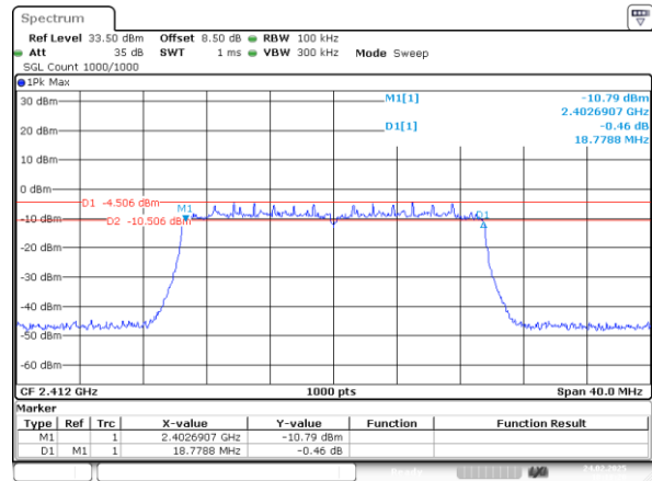
802.11ax20_2412MHz_Chain 1
