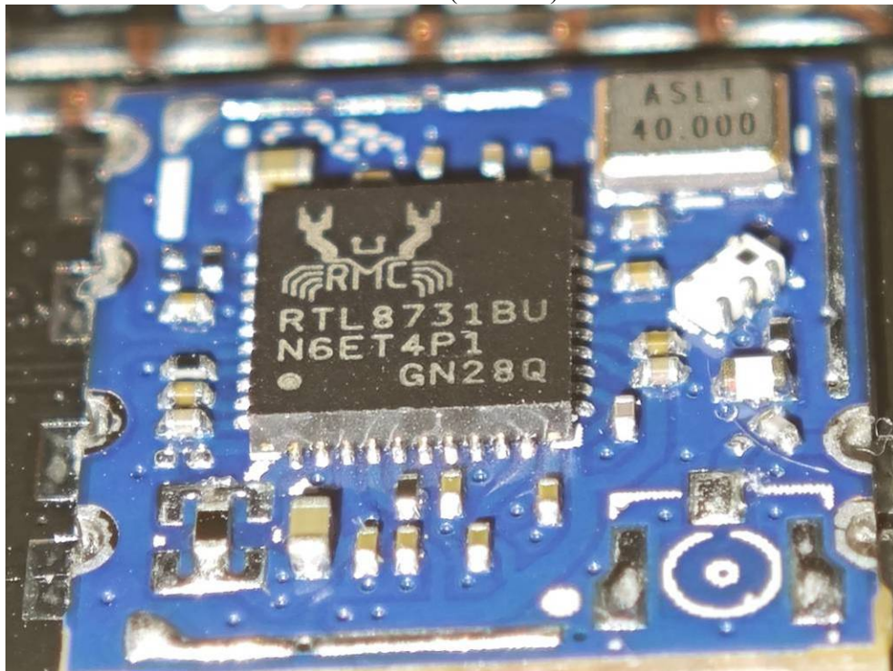
Module 1(2.4G/5G)
