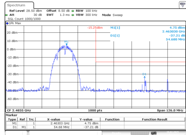
802.11b_2462MHz_Chain 0
