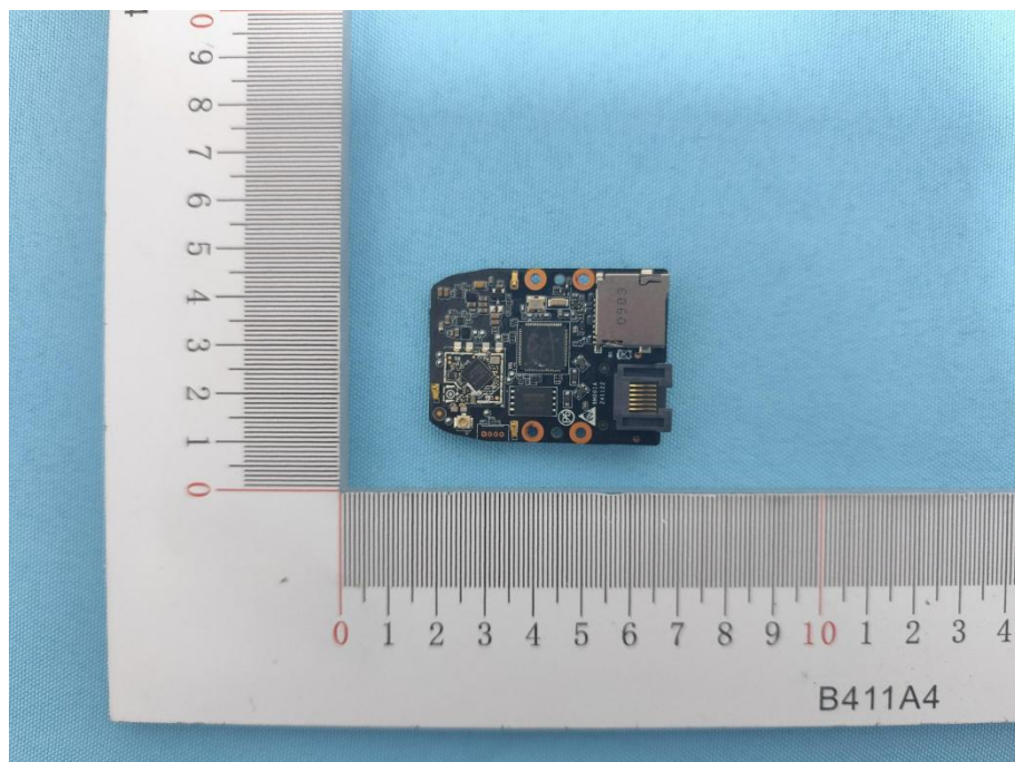
SRD ANT
