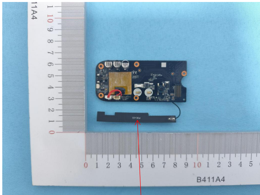
SRD ANT
