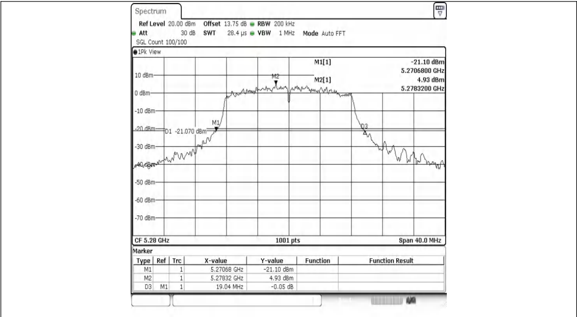
802.11a-Ant1-5280
