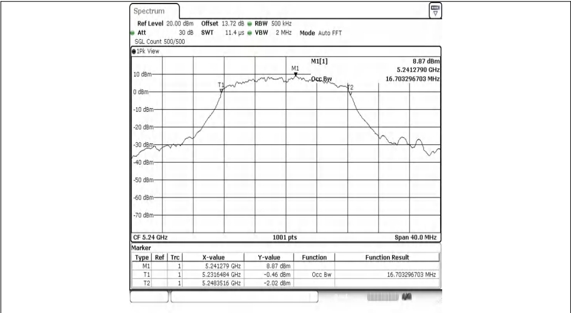
802.11a-Ant1-5240
