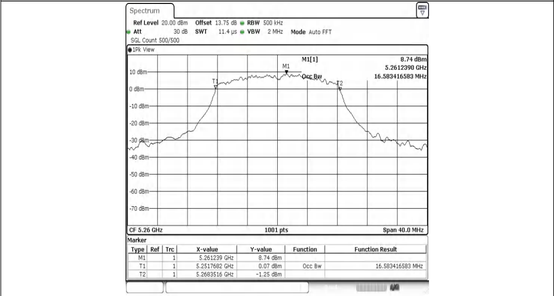
802.11a-Ant1-5260
