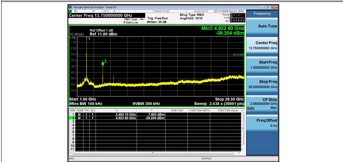
802.11b-Ant1-2462-1000~26500-PASS
