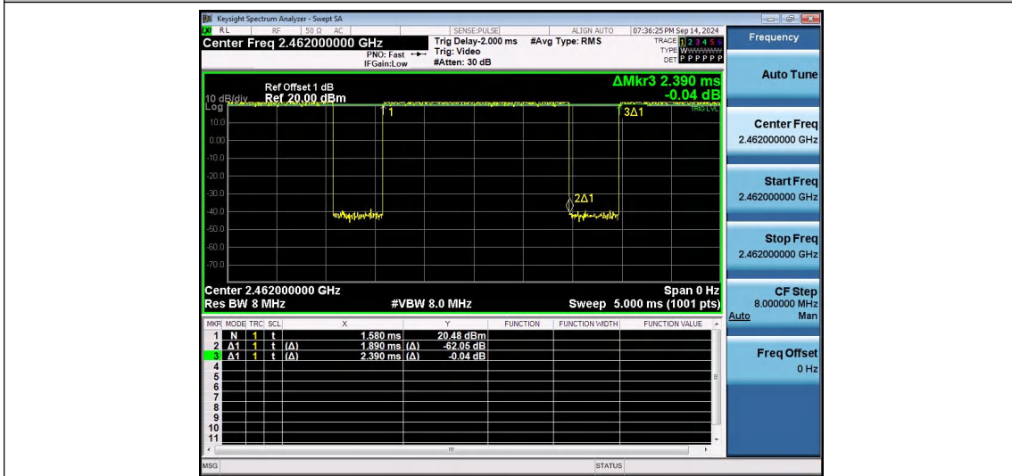
NTNV-802.11n(HT20)SISO-Ant1-2462
