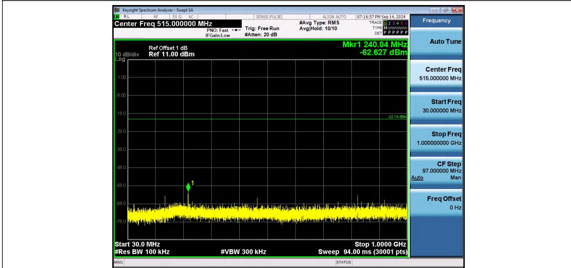
802.11b-Ant1-2462-30~1000-PASS
