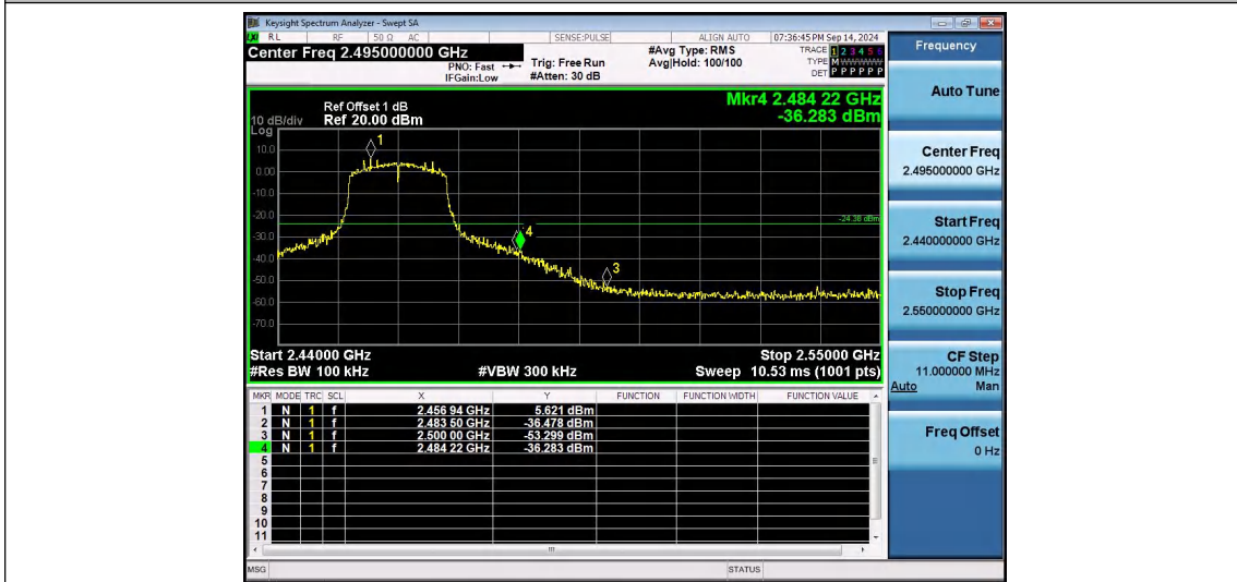
802.11n-HT20)SISO-Ant1-2462-PASS
