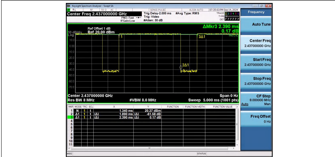
NTNV-802.11n(HT20)SISO-Ant1-2437
