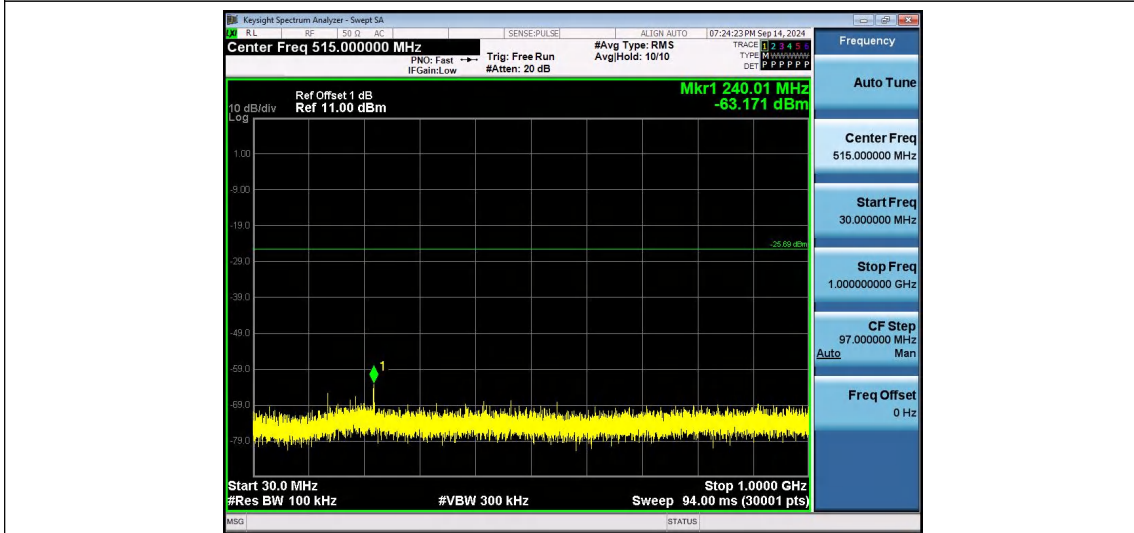
802.11g-Ant1-2437-30~1000-PASS
