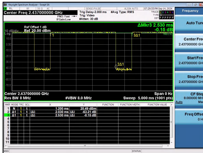
NTNV-802.11g-Ant1-2437
