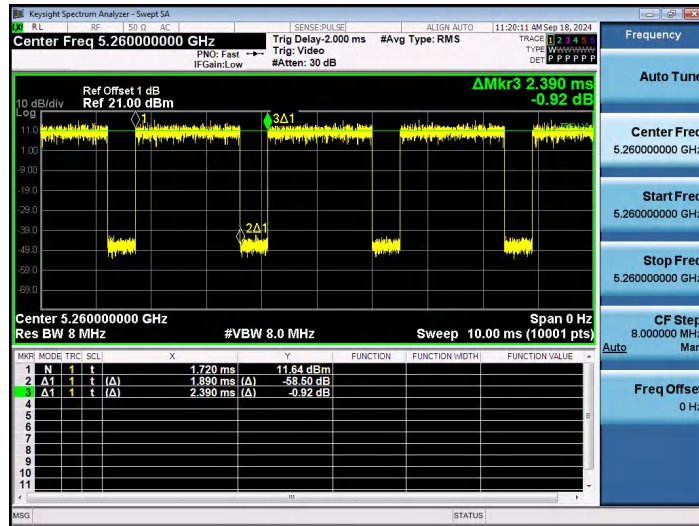
NTNV-802.11n(HT20)SISO-Ant1-5260
