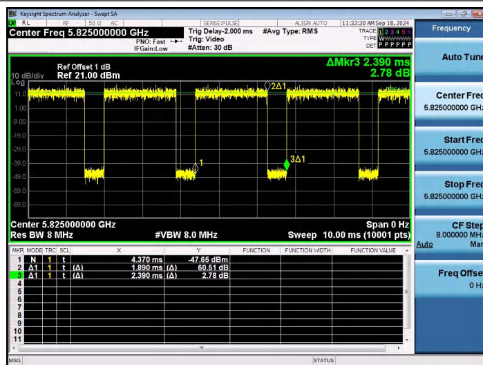
NTNV-802.11n(HT20)SISO-Ant1-5825
