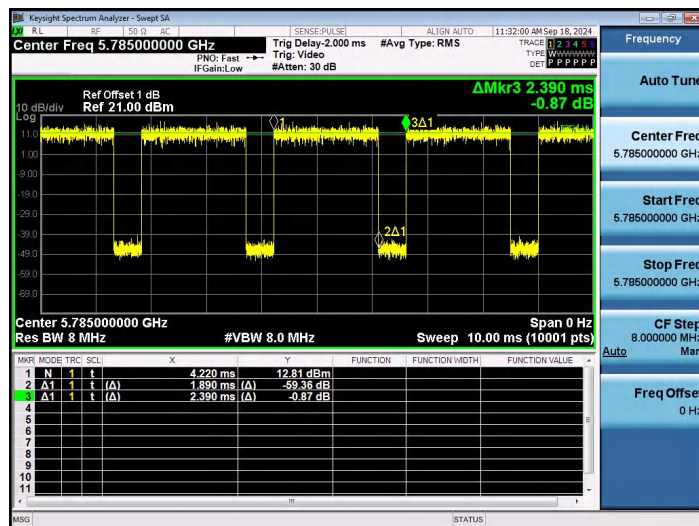
NTNV-802.11n(HT20)SISO-Ant1-5785
