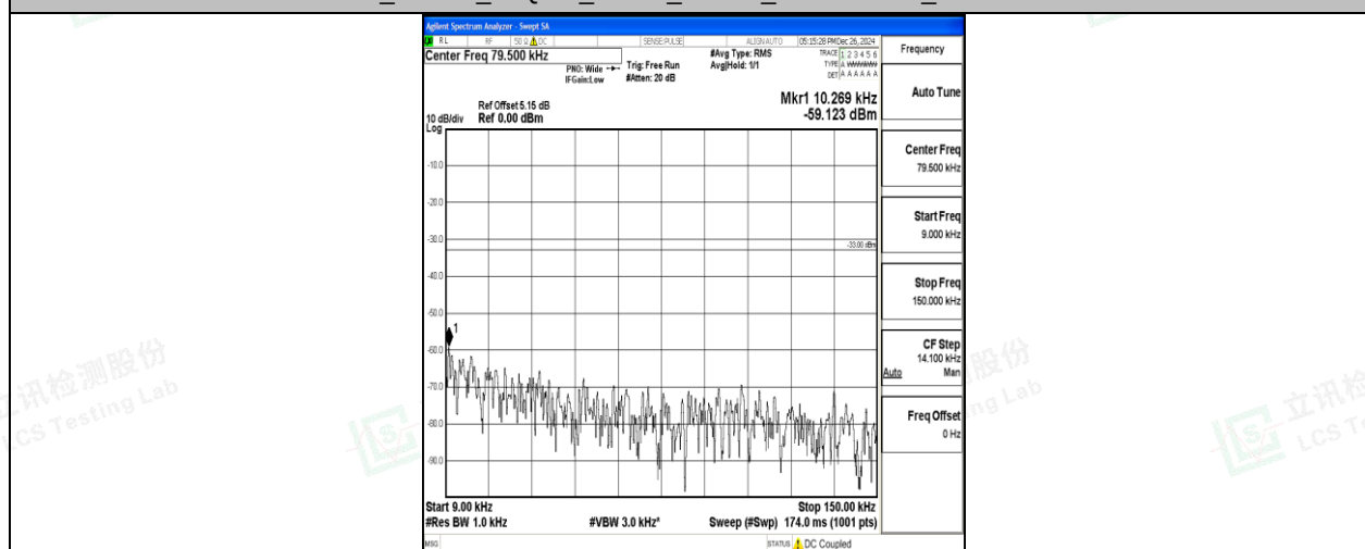
Band5 10MHz QPSK 20525 1RB#0 0.009~0.15 0.009~0.15
