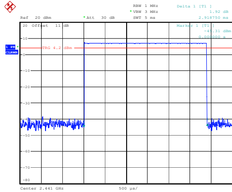
DH5_Hopping 2.919ms
