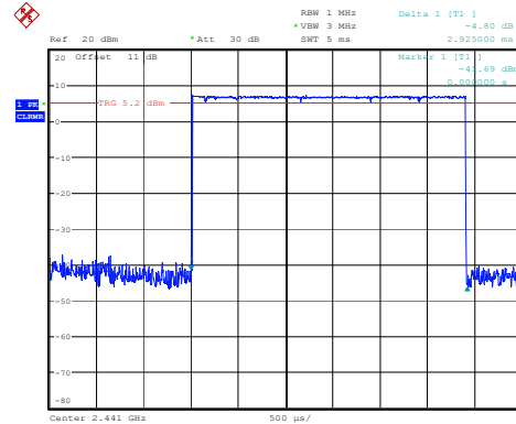
2DH5_Hopping 2.925ms
