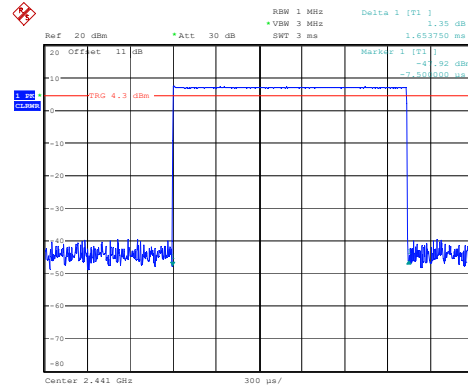
DH3_Hopping 1.654ms
