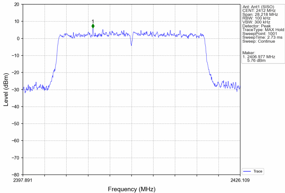
802.11ax(HEW20)_LCH_2412MHz_SU_/_Ant1 (SISO)_NTNV
