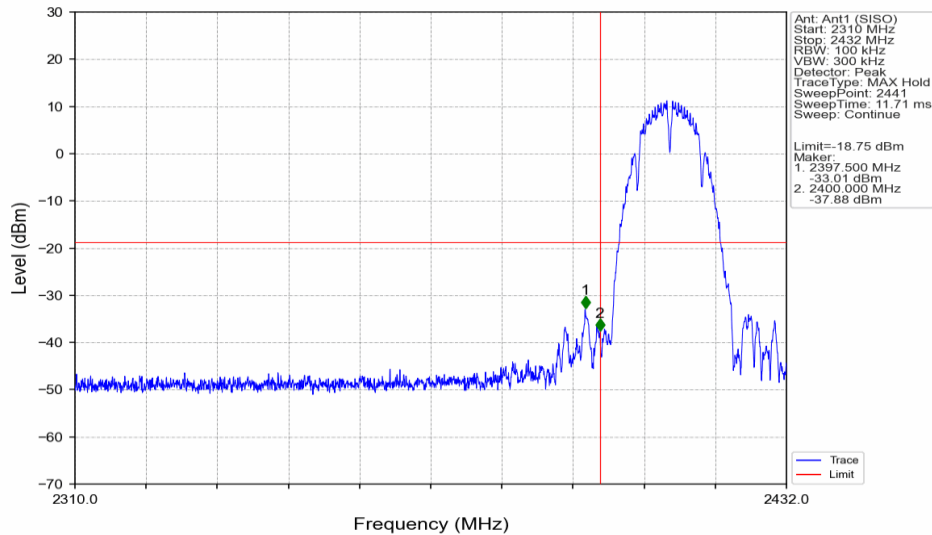
802.11b_LCH_2412MHz_Ant1 (SISO)_NTNV
