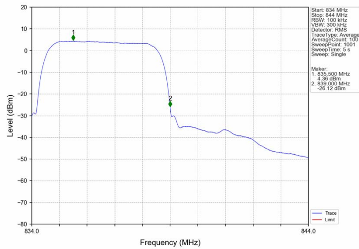
Band5_HSUPA_MCH_836.6MHz_Subtest 1_NTNV
