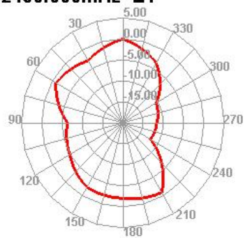
2450.000MHz E1
