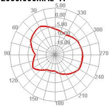
2500.000MHz H
