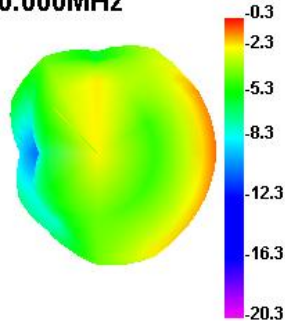
2400.000MHz
