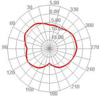
2450.000MHz H
