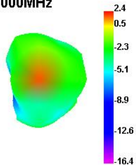
2500.000MHz
