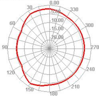
2400.000MHz E2
