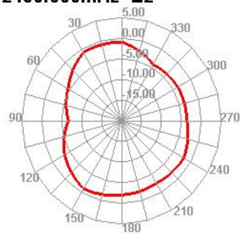
2450.000MHz E2
