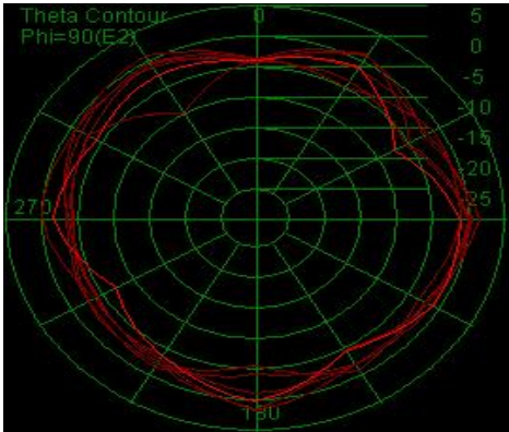
V YZ轴 2450MHz
