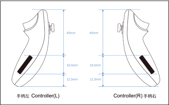
贴纸位置
