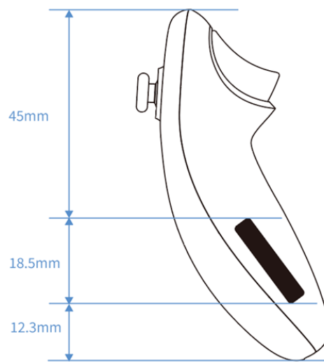
手柄右
