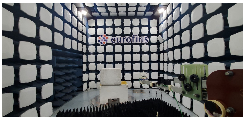
18GHz - 26.5GHz
