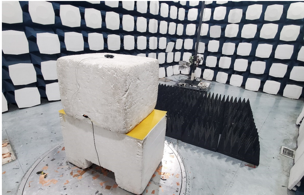
1GHz-18GHz
