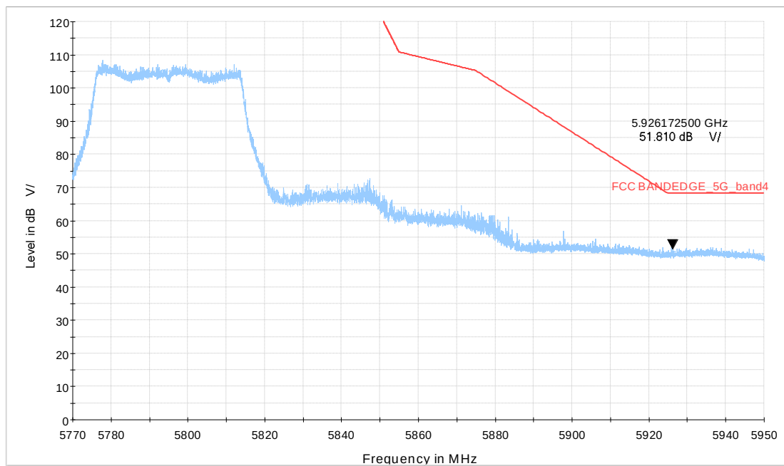
Wi-Fi 5GHz_BE40 CH159
