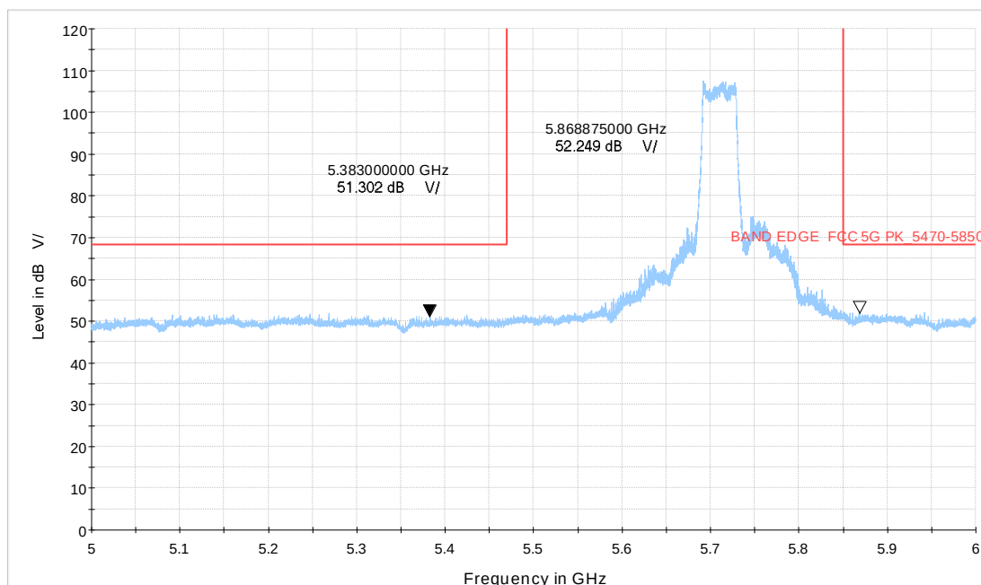
Wi-Fi 5GHz_BE40 CH142
