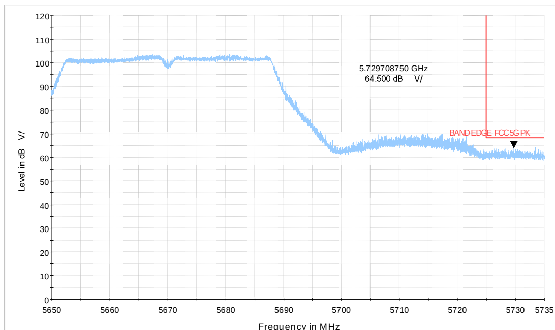
Wi-Fi 5GHz_n40 CH134
