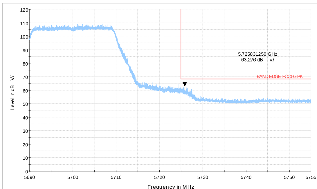
Wi-Fi 5GHz_BE20 CH140
