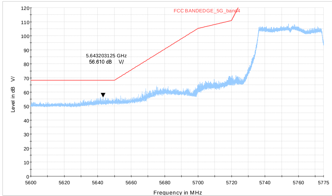
Wi-Fi 5GHz_BE40 CH151
