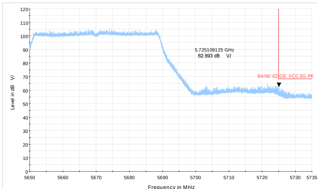
Wi-Fi 5GHz_BE40 CH134
