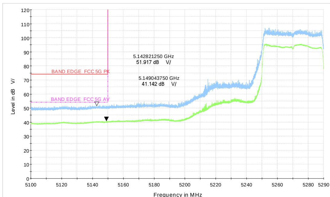
Wi-Fi 5GHz_BE40 CH54
