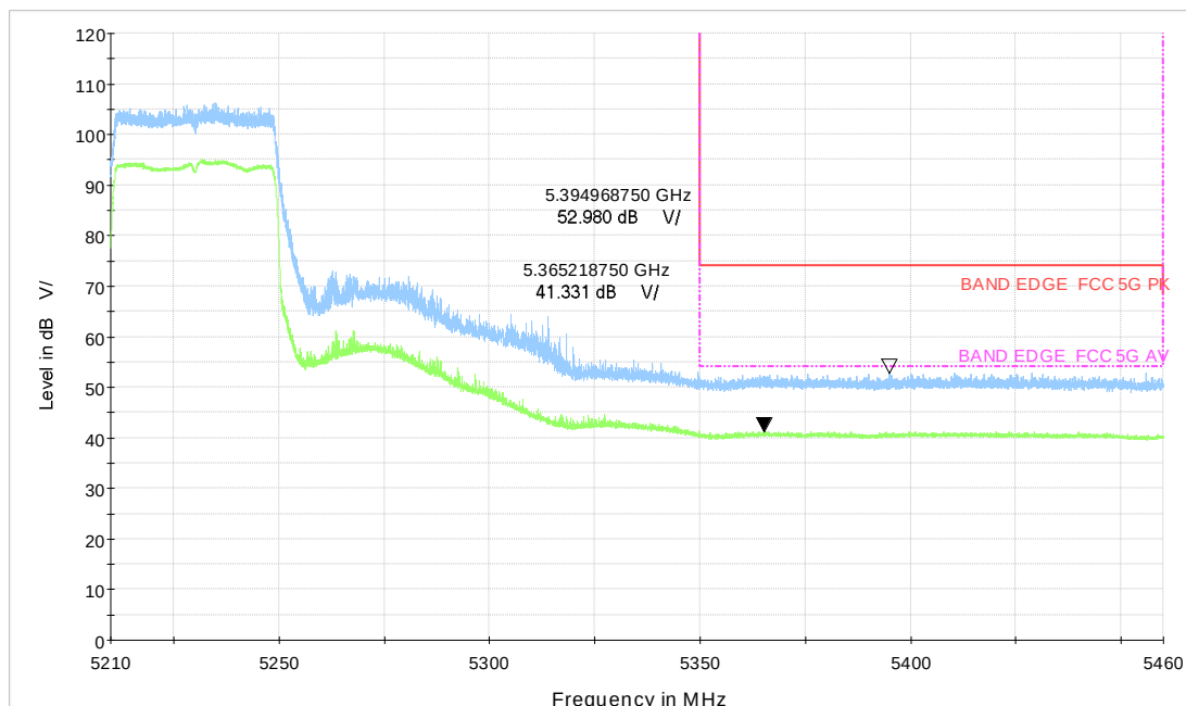
Wi-Fi 5GHz_BE40 CH46
