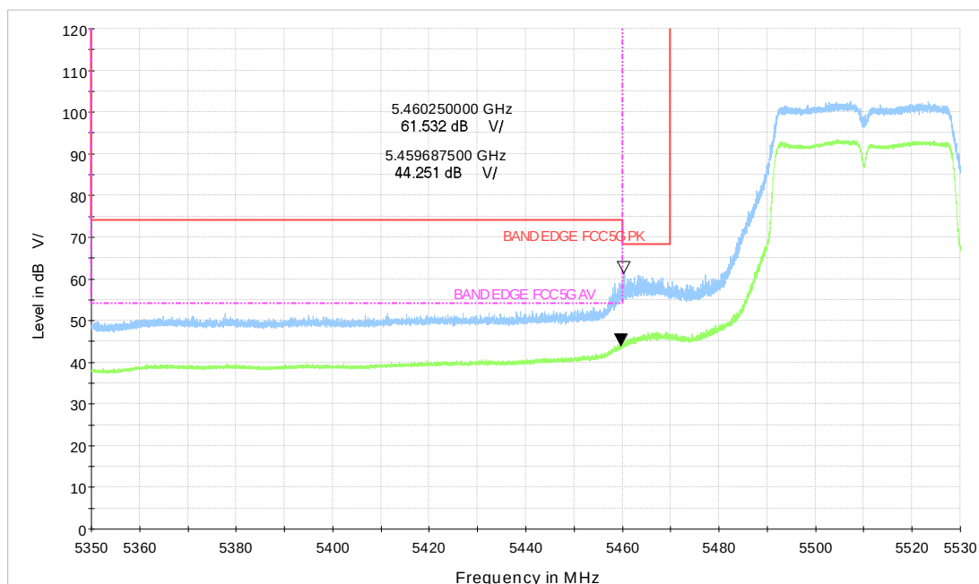
Wi-Fi 5GHz_n40 CH102
