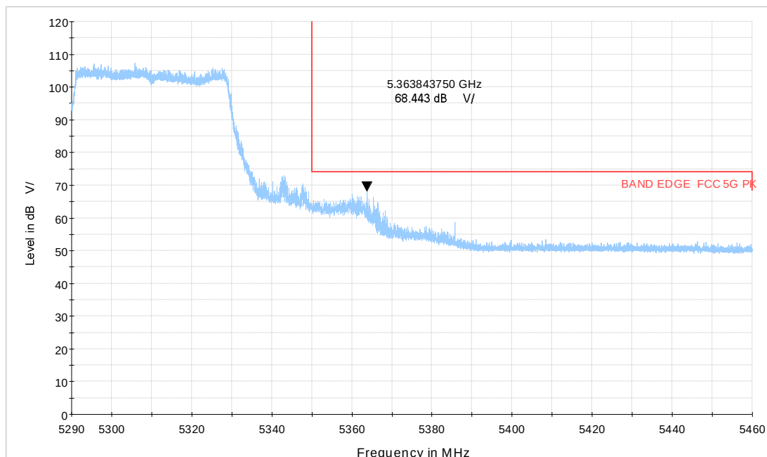
Wi-Fi 5GHz_BE40 CH62
