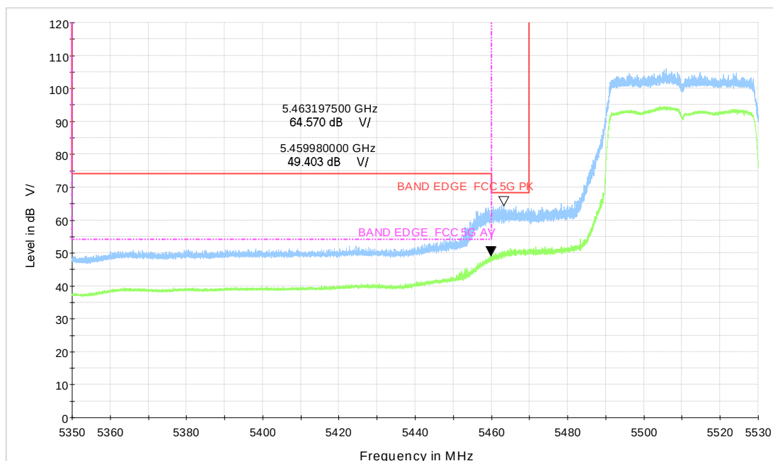
Wi-Fi 5GHz_BE40 CH102
