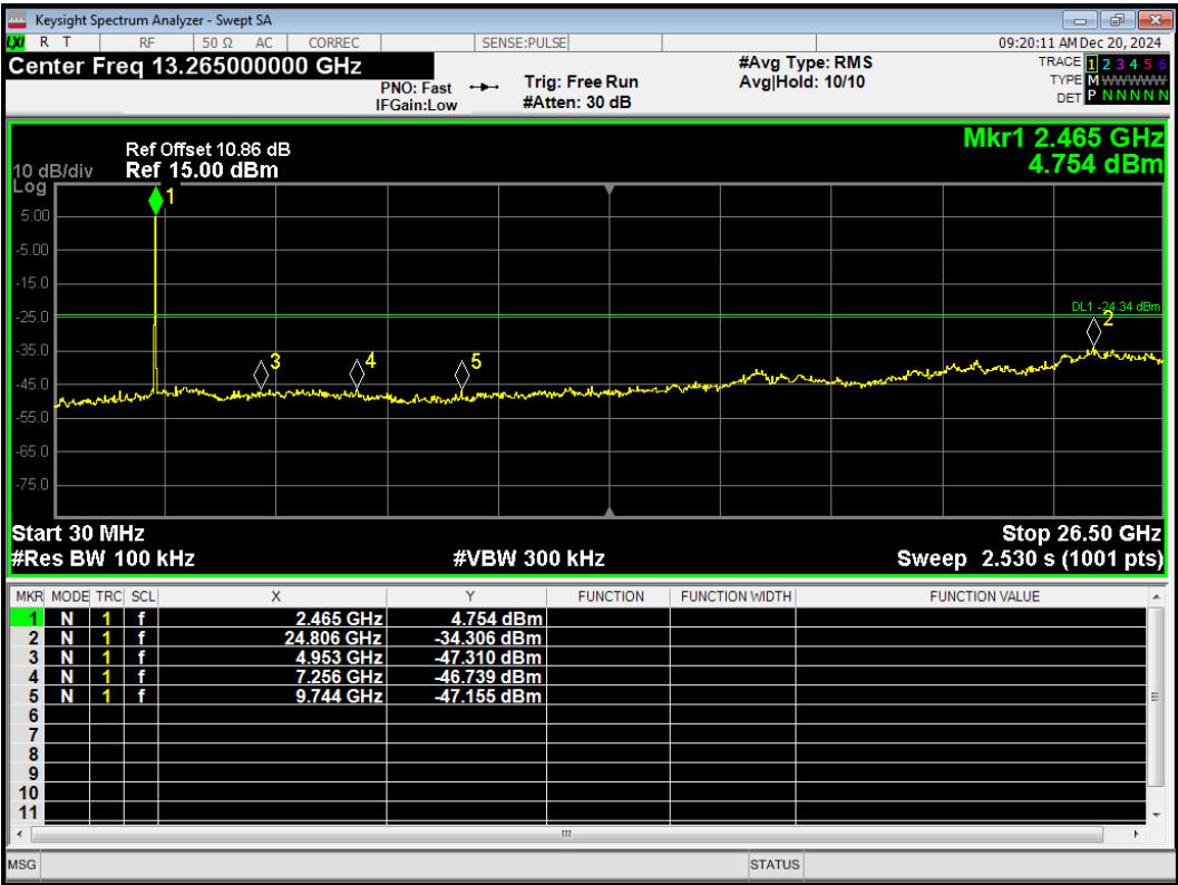
Tx. Spurious 802.11be(40) 484-Tones Index65 2422MHz Ref
