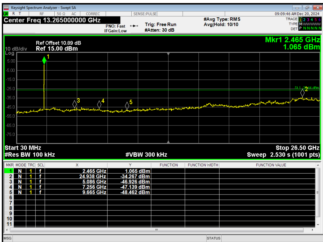
Tx. Spurious 802.11be(20) 52-Tones Index40 2462MHz Ref
