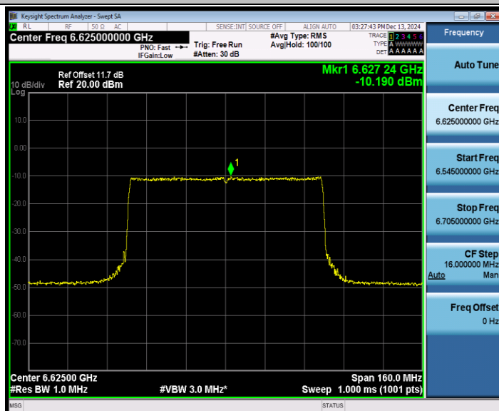
802.11be 80 MIMO_Ant2_6625
