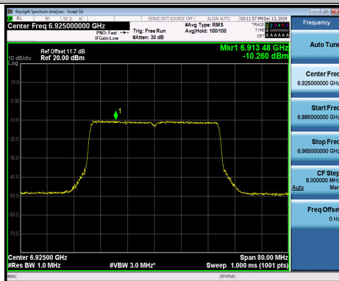
802.11be 40 MIMO_Ant2_6925
