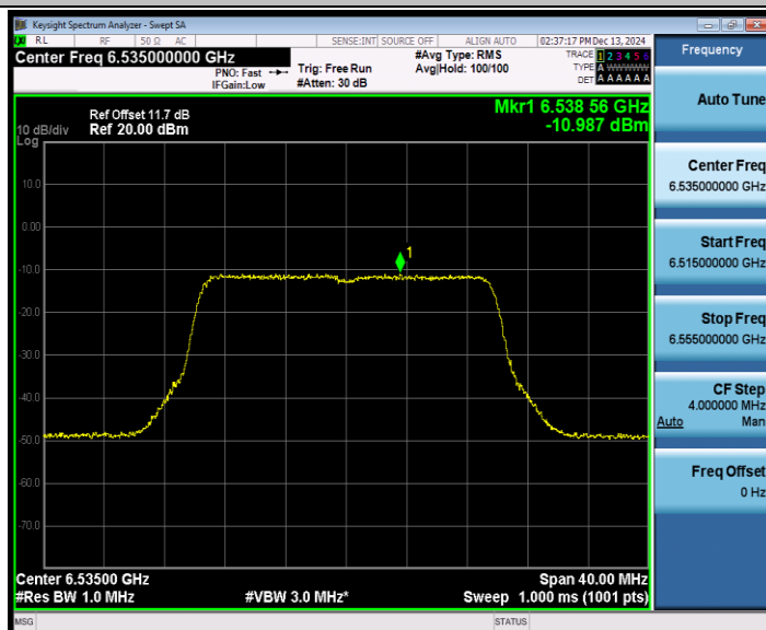
802.11be 20 MIMO_Ant2_6535
