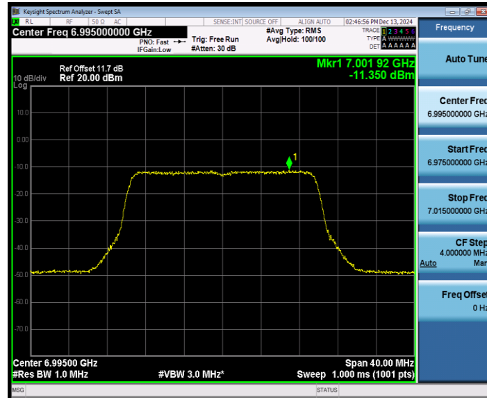
802.11be 20 MIMO_Ant2_6995
