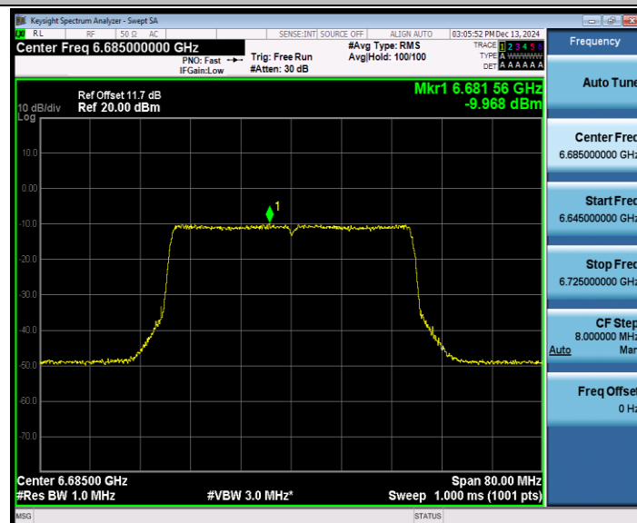
802.11be 40 MIMO_Ant2_6685
