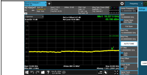
Band41(2555-2655)-10MHz-QPSK-40190-50RB#0-30-1000-PASS
