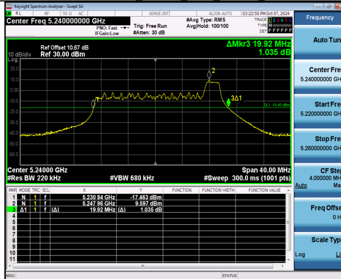
11AX20MIMO Ant W1 5240 52Tone RU40
