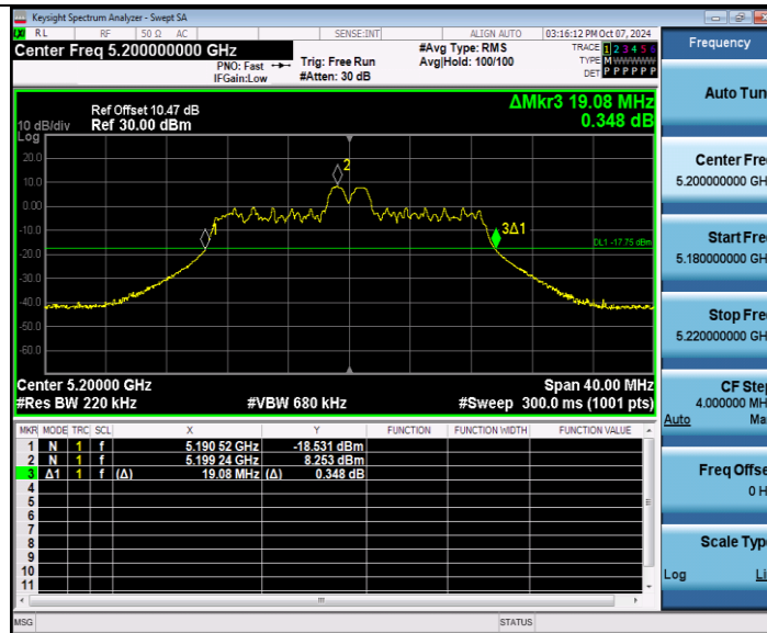
11AX20MIMO_Ant W0_5200_52Tone_RU38
