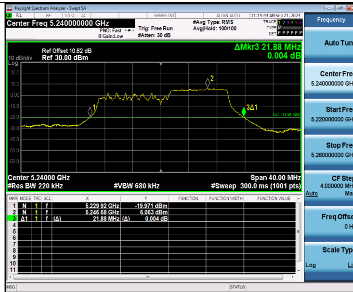
11AX20MIMO Ant W1 5240 26Tone RU8
