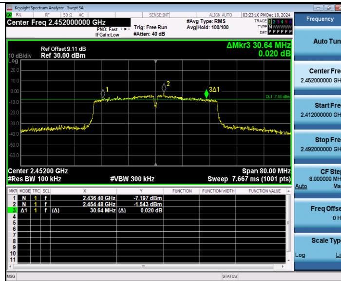
11N40MIMO_Ant W1_2452
