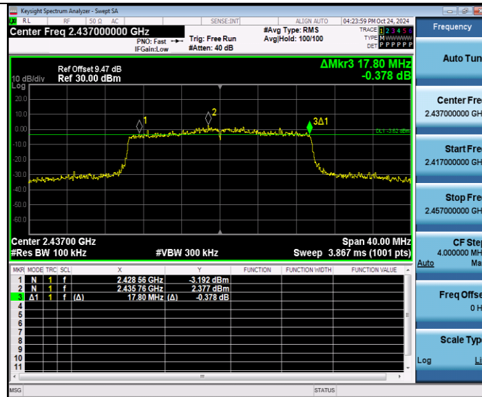
11AX20MIMO_Ant W1_2437
