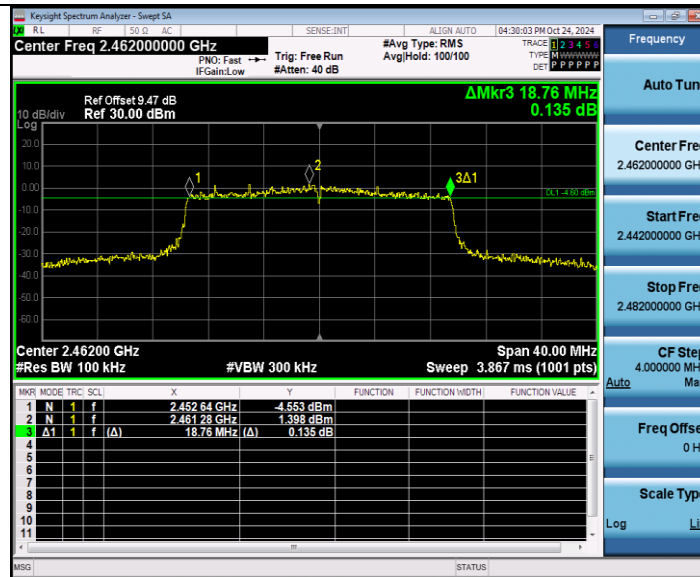
11AX20MIMO_Ant W1_2462
