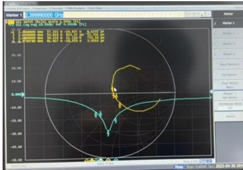
Vibetag-PCB-V1.0 调试效果图
