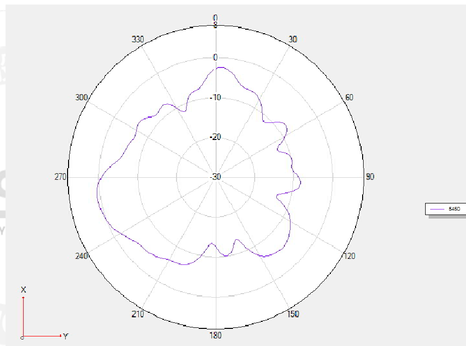
5450MHz @ \Theta:90^\circ
