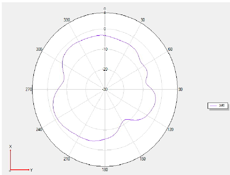
2450MHz @ \Theta:90^\circ
