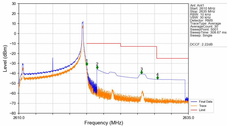
Band38_10MHz_QPSK_HCH_2615MHz_RB_1_49_NTNV
