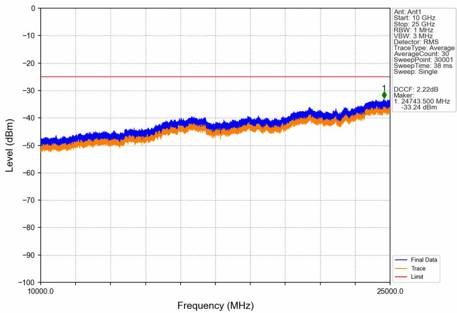
Band38_10MHz_QPSK_HCH_2615MHz_RB_1_0_NTNV
