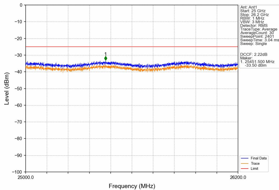
Band38_10MHz_QPSK_MCH_2595MHz_RB_1_0_NTNV
