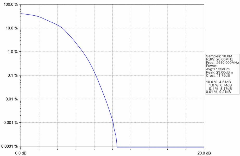
Band38_20MHz_16QAM_HCH_2610MHz_RB_100_0_NTNV
