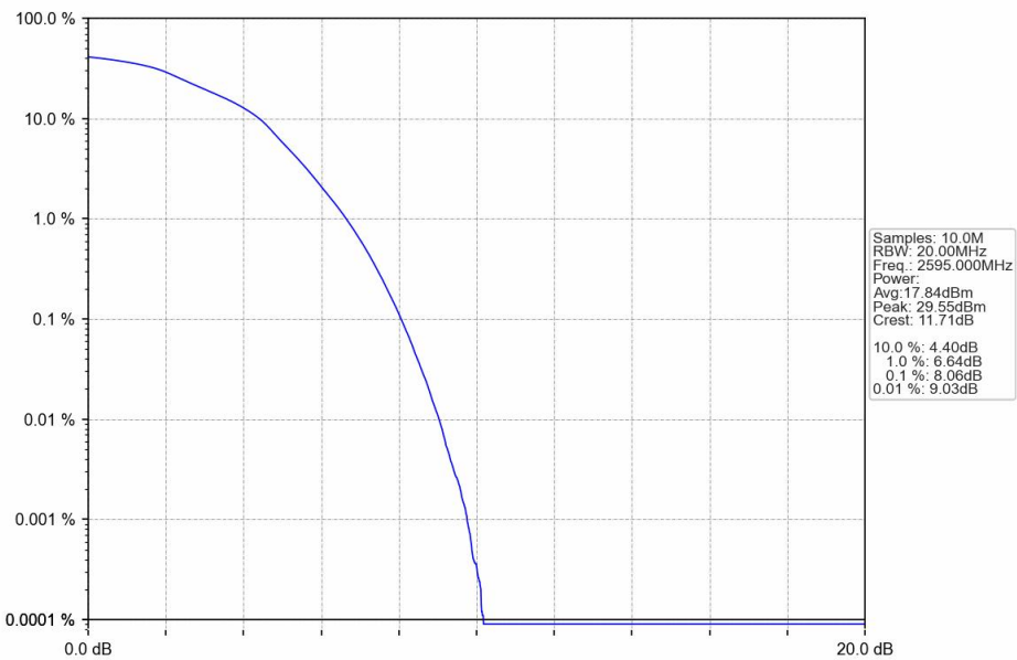
Band38_20MHz_16QAM_MCH_2595MHz_RB_100_0_NTNV
