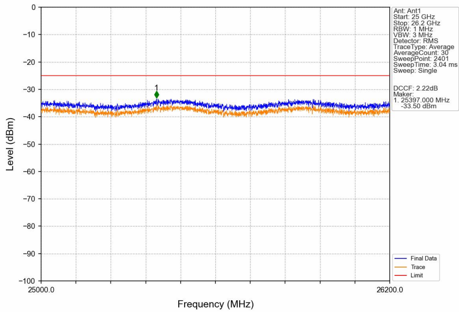
Band38_10MHz_QPSK_HCH_2615MHz_RB_1_49_NTNV
