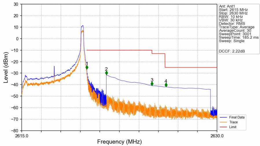
Band38_5MHz_QPSK_HCH_2617.5MHz_RB_1_24_NTNV
