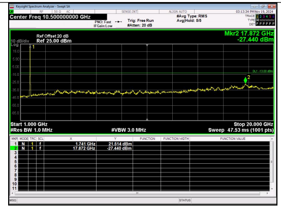
1000.0MHz-20000.0MHz Band 66 10MHz/1745.0/Mid QPSK 1@0
