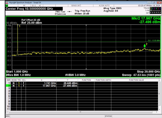
1000.0MHz-20000.0MHz Band 66 15MHz/1745.0/Mid QPSK 1@0
