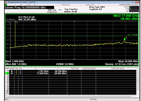
1000.0MHz-20000.0MHz Band 66 5MHz/1745.0/Mid QPSK 1@0
