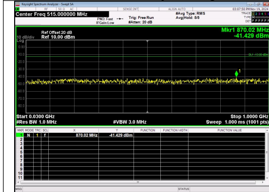
30.0MHz-1000.0MHz Band 66 5MHz/1745.0/Mid QPSK 1@0
