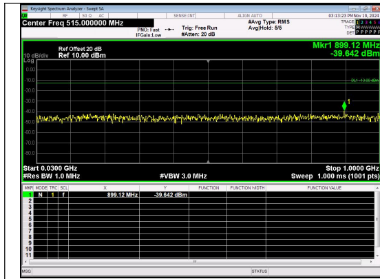
30.0MHz-1000.0MHz Band 66 10MHz/1745.0/Mid QPSK 1@0
