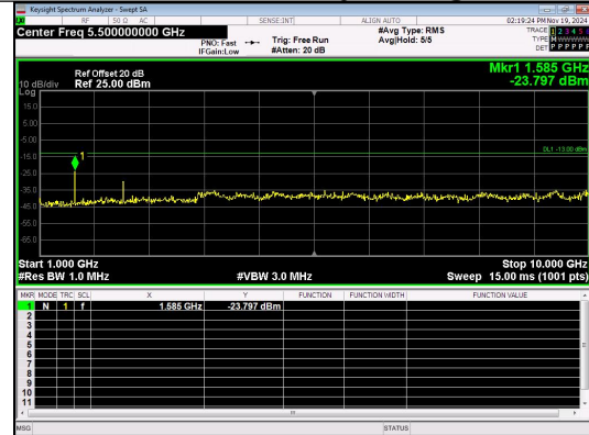
1000.0MHz-10000.0MHz Band 14 5MHz/793.0/Mid QPSK 1@0
