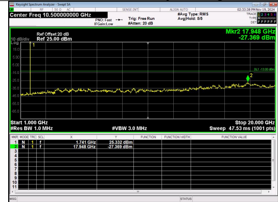
1000.0MHz-20000.0MHz Band 66 1.4MHz/1745.0/Mid QPSK 1@0
