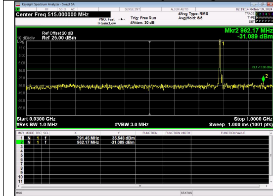
30.0MHz-1000.0MHz Band 14 5MHz/793.0/Mid QPSK 1@0
