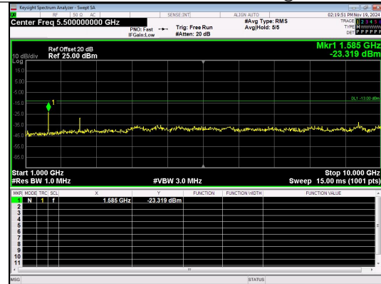
1000.0MHz-10000.0MHz Band 14 5MHz/793.0/Mid 16QAM 1@0
