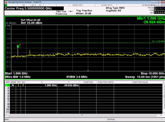
1000.0MHz-10000.0MHz Band 12 5MHz/701.5/Low 16QAM 1@0
