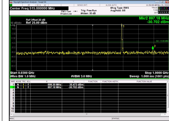
30.0MHz-1000.0MHz Band 12 5MHz/701.5/Low 16QAM 1@0
