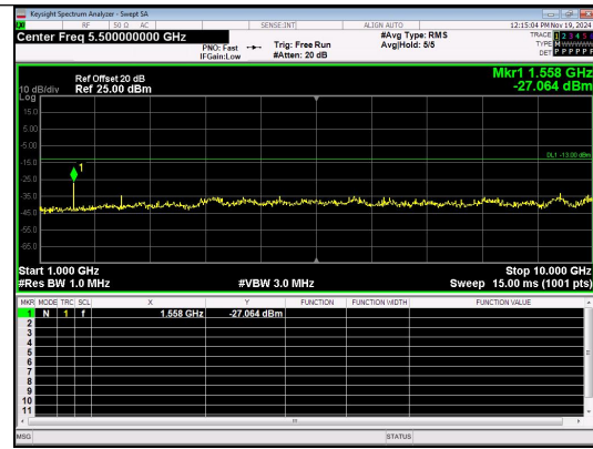
1000.0MHz-10000.0MHz Band 13 10MHz/782.0/Mid QPSK 1@0
