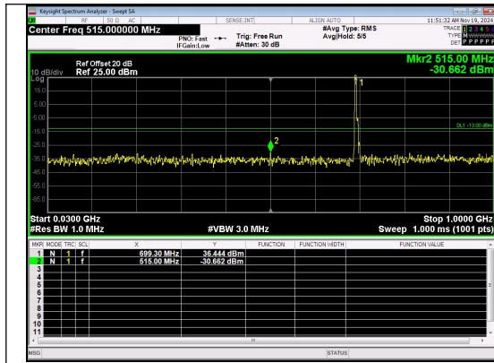
30.0MHz-1000.0MHz Band 12 5MHz/701.5/Low QPSK 1@0
