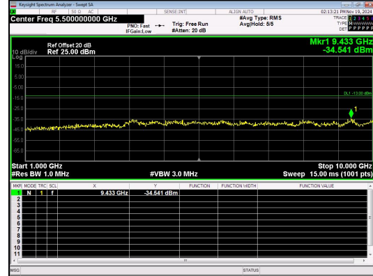
1000.0MHz-10000.0MHz Band 13 10MHz/782.0/Mid 16QAM 1@0
