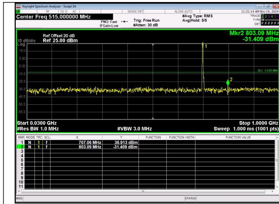
30.0MHz-1000.0MHz Band 12 3MHz/707.5/Mid QPSK 1@0
