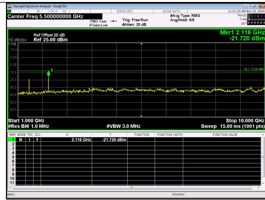
1000.0MHz-10000.0MHz Band 12 3MHz/707.5/Mid QPSK 1@0
