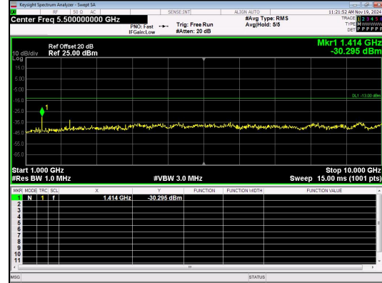
1000.0MHz-10000.0MHz Band 12 3MHz/707.5/Mid 16QAM 1@0
