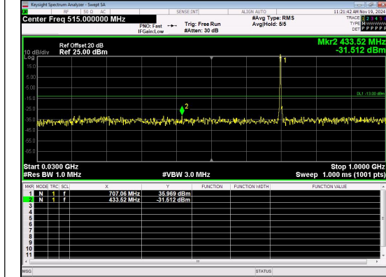
30.0MHz-1000.0MHz Band 12 3MHz/707.5/Mid 16QAM 1@0
