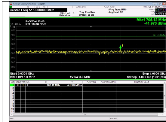
30.0MHz-1000.0MHz Band 4 10MHz/1732.5/Mid QPSK 1@0
