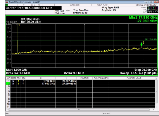
1000.0MHz-20000.0MHz Band 4 20MHz/1732.5/Mid QPSK 1@0
