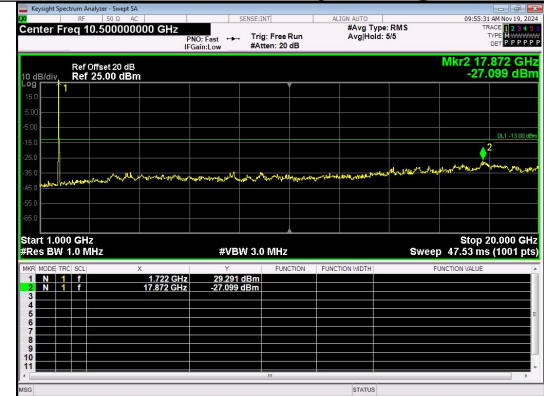
1000.0MHz-20000.0MHz Band 4 15MHz/1732.5/Mid QPSK 1@0
