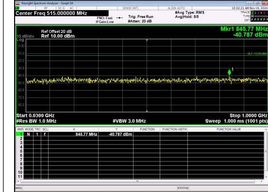
30.0MHz-1000.0MHz Band 4 20MHz/1732.5/Mid QPSK 1@0
