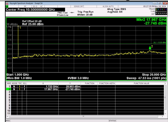
1000.0MHz-20000.0MHz Band 4 15MHz/1732.5/Mid 16QAM 1@0
