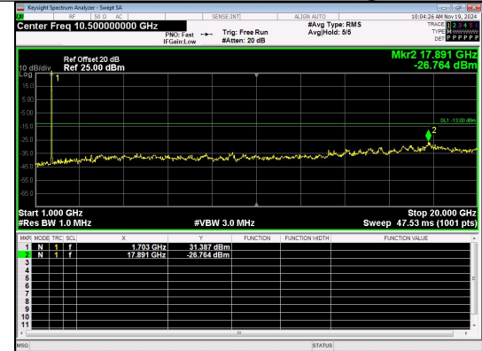
1000.0MHz-20000.0MHz Band 4 20MHz/1720.0/Low QPSK 1@0
