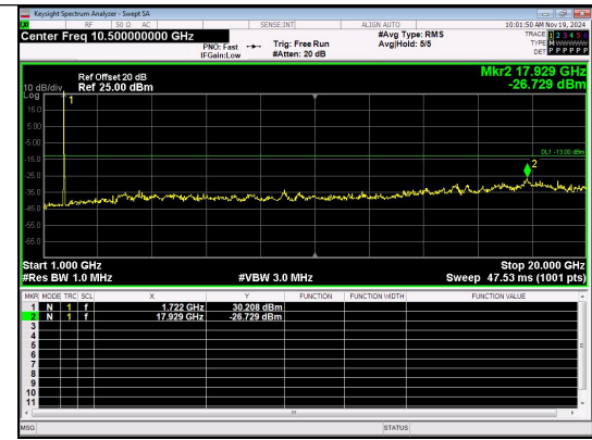
1000.0MHz-20000.0MHz Band 4 20MHz/1732.5/Mid QPSK 1@0
