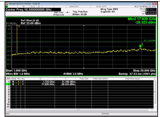
1000.0MHz-20000.0MHz Band 4 10MHz/1732.5/Mid QPSK 1@0
