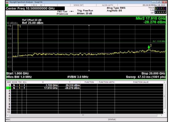
1000.0MHz-20000.0MHz Band 4 10MHz/1732.5/Mid 16QAM 1@0
