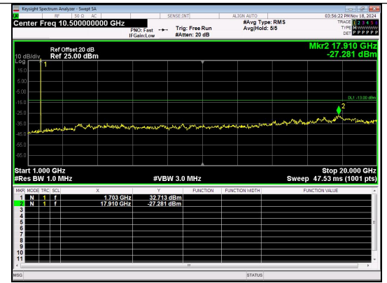
1000.0MHz-20000.0MHz Band 4 1.4MHz/1710.7/Low QPSK 1@0
