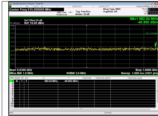
30.0MHz-1000.0MHz Band 2 20MHz/1880.0/Mid QPSK 1@0
