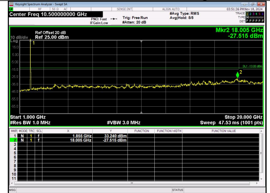
1000.0MHz-20000.0MHz Band 2 20MHz/1880.0/Mid 16QAM 1@0
