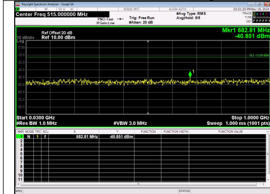
30.0MHz-1000.0MHz Band 2 20MHz/1880.0/Mid 16QAM 1@0
