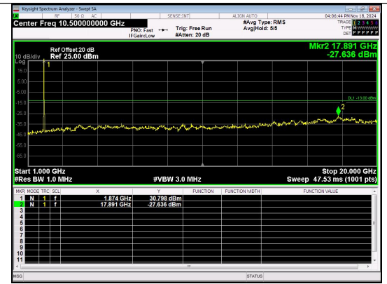
1000.0MHz-20000.0MHz Band 2 20MHz/1880.0/Mid QPSK 1@0
