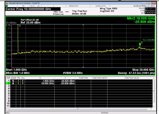
1000.0MHz-20000.0MHz Band 2 20MHz/1860.0/Low QPSK 1@0
