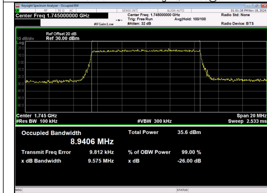
Band 66 10MHz/1745.0/Mid QPSK 50@0
