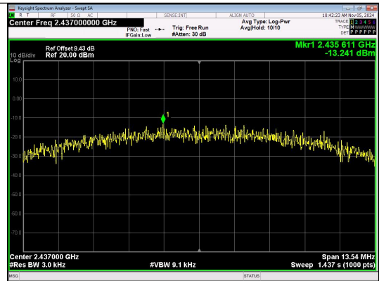
IEEE 802.11b_Channel 6_20MHz_Antenna 2
