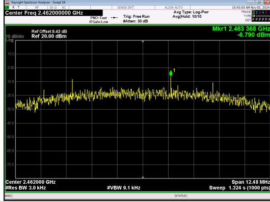
IEEE 802.11b_Channel 11_20MHz_Antenna 2
