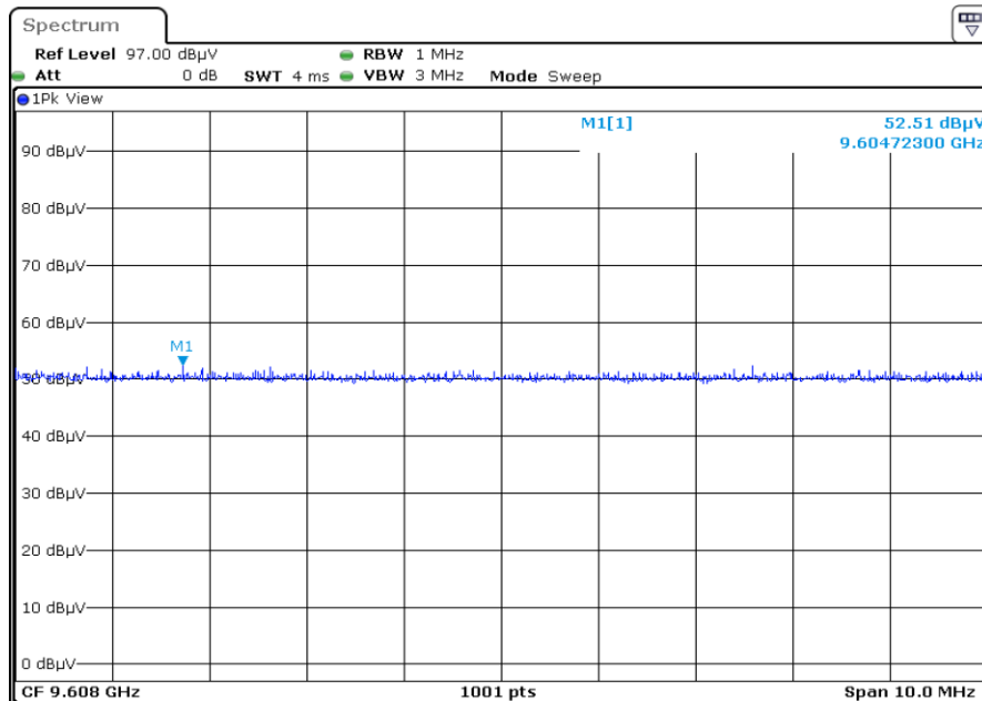
F1 X4 9608.0 Harmonic Horizontal PEAK
