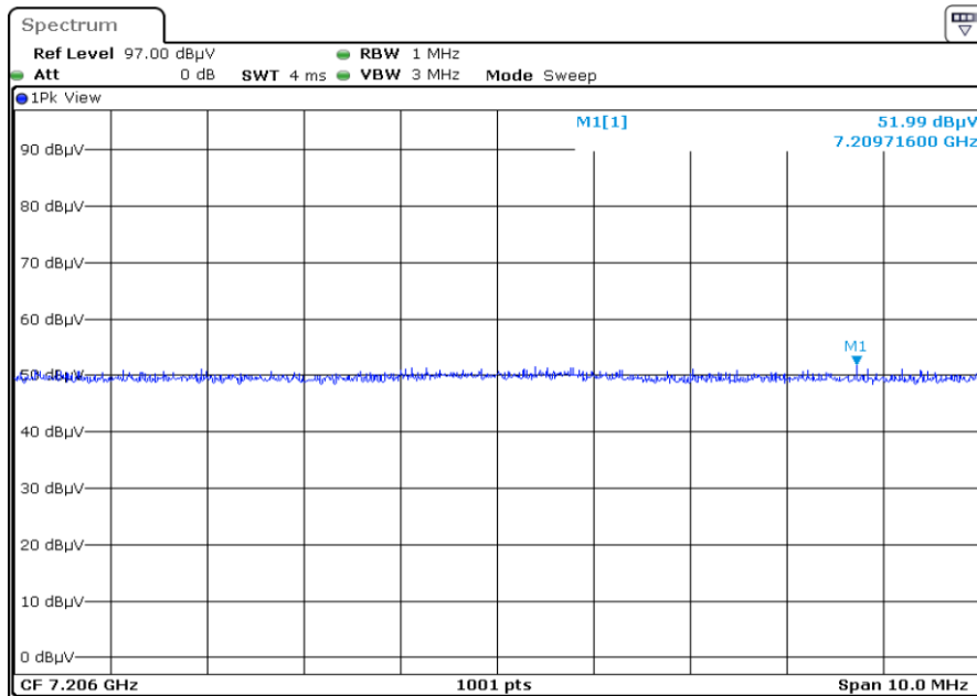
F1 X3 7206.0 Harmonic Horizontal PEAK
