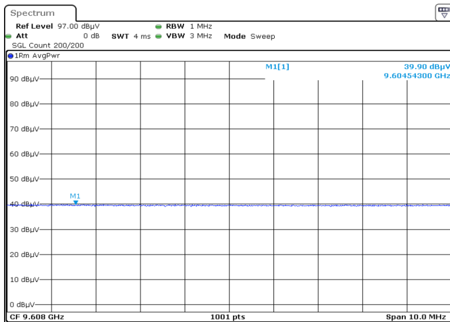
F1 X4 9608.0 Harmonic Horizontal AVG
