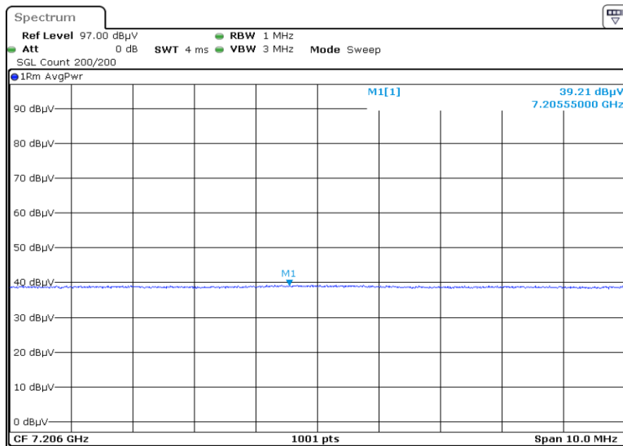
F1 X3 7206.0 Harmonic Horizontal AVG
