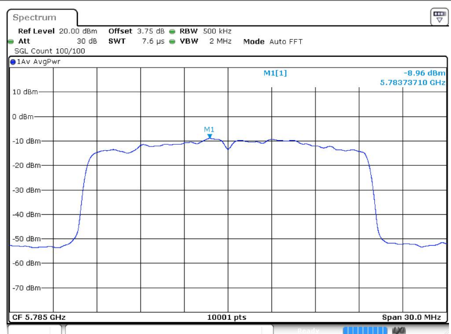
PSD ax20 5785MHz Ant1
