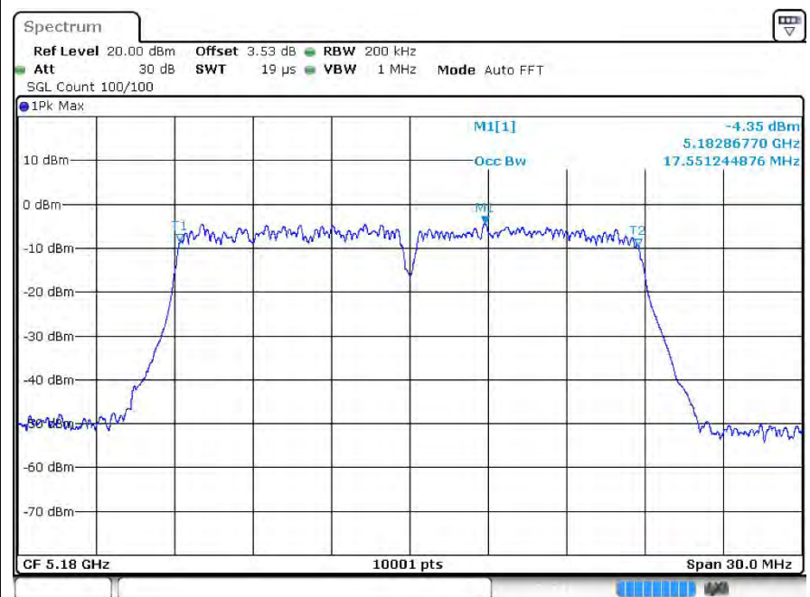
OBW n20 5180MHz Ant2
