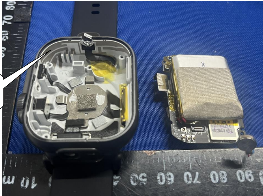
LTE antenna
