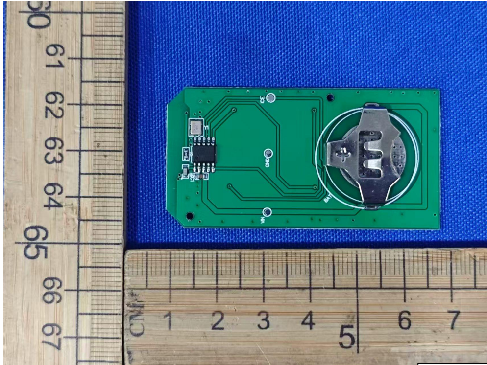
2.4G ANT
