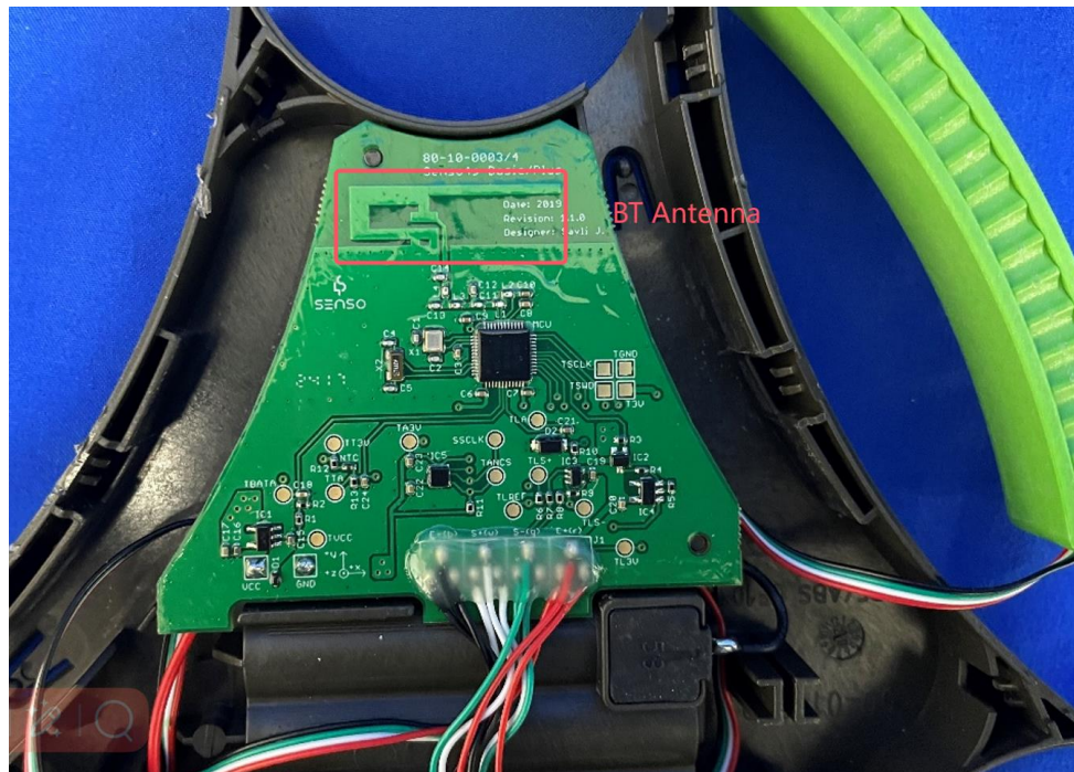
(18) EUT Photo (PLUS)
