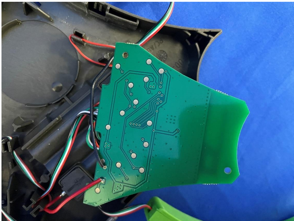
(18) EUT Photo (PLUS)
