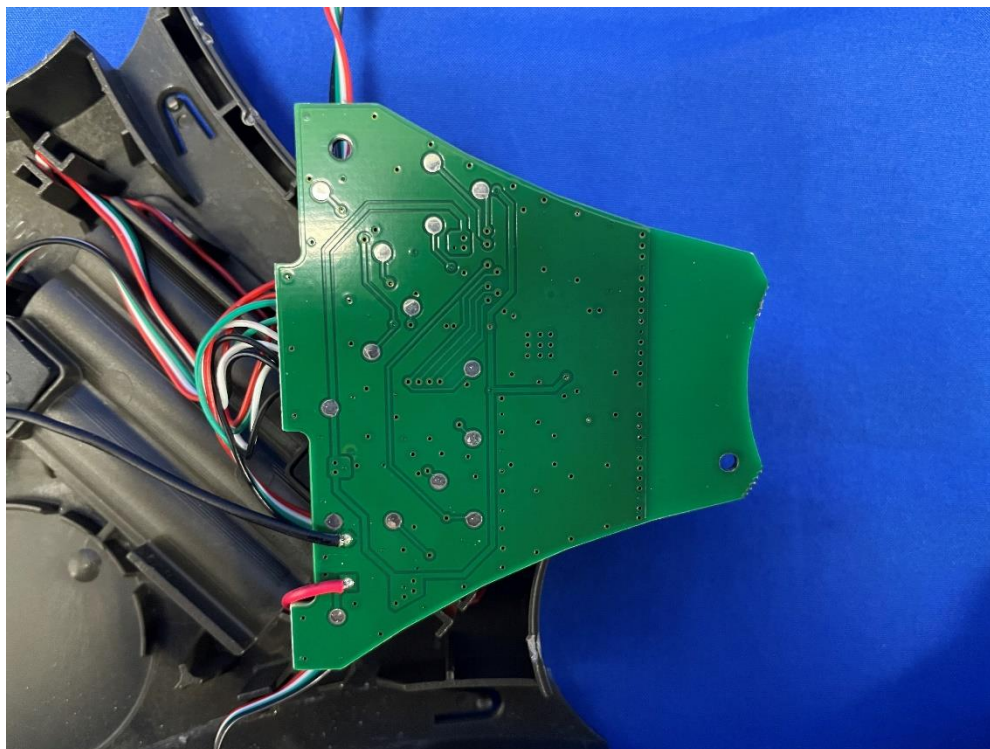
(14) EUT Photo (PLUS)
