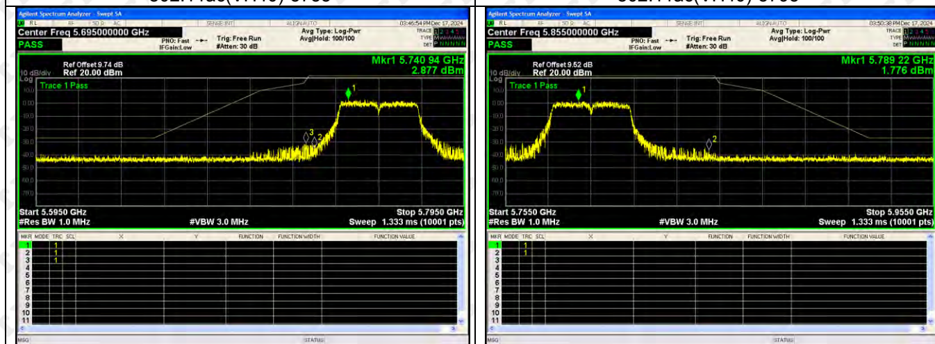
802.11(n20)-5745
