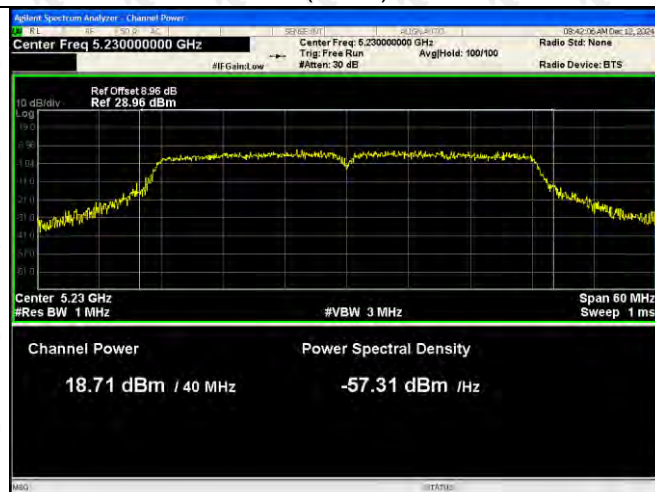
802.11n(VH40)-5230
