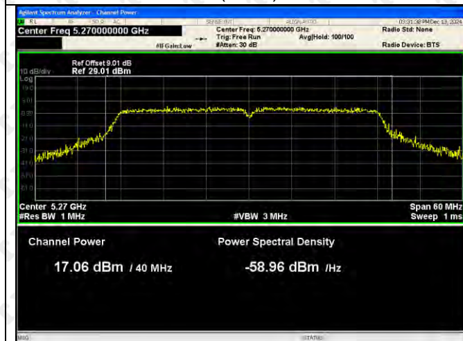
802.11n(VH40)-5270
