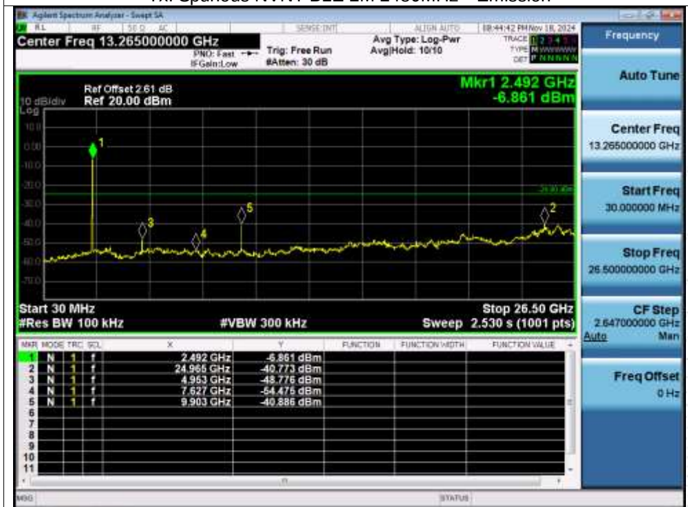
Tx. Spurious NVNT BLE 2M 2480MHz Emission
