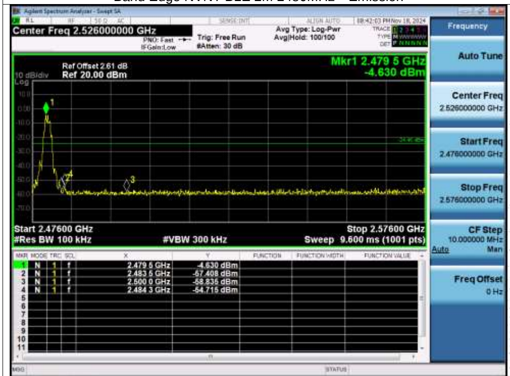
Band Edge NVNT BLE 2M 2480MHz Emission
