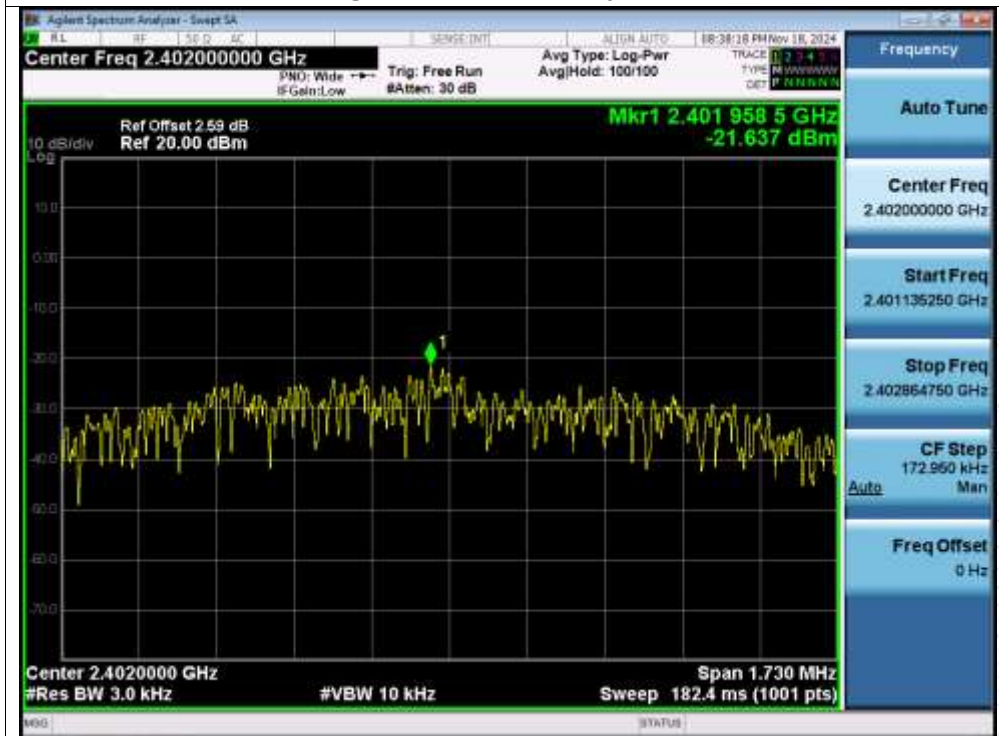
PSD NVNT BLE 2M 2402MHz
