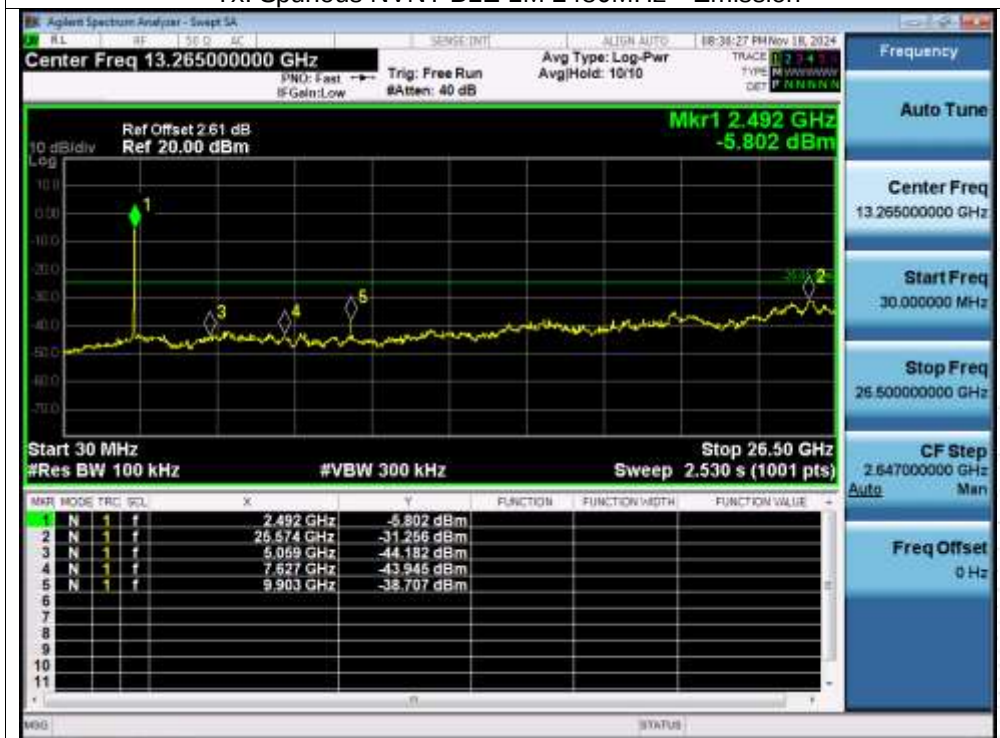
Tx. Spurious NVNT BLE 1M 2480MHz Emission
