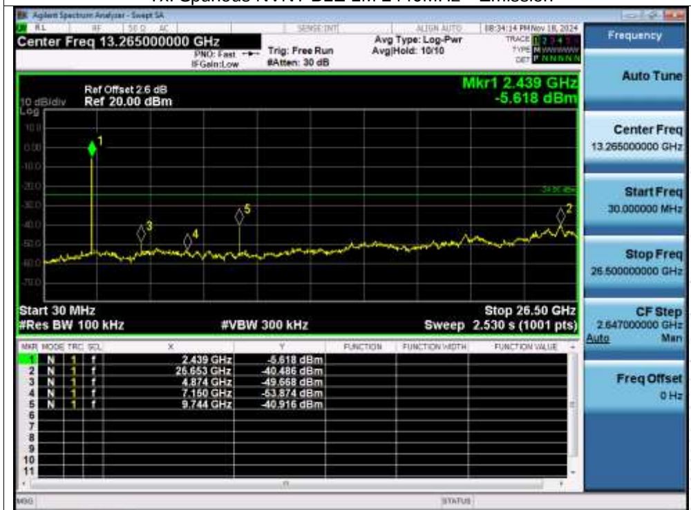
Tx. Spurious NVNT BLE 1M 2440MHz Emission
