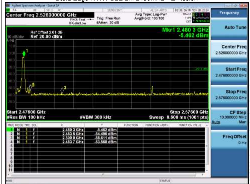
Band Edge NVNT BLE 1M 2480MHz Emission
