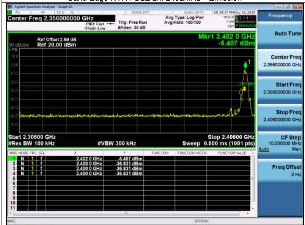
Band Edge NVNT BLE 2M 2402MHz Emission
