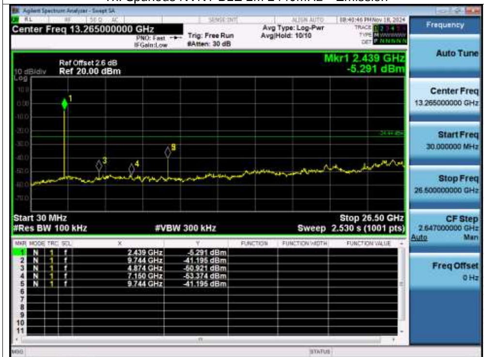
Tx. Spurious NVNT BLE 2M 2440MHz Emission
