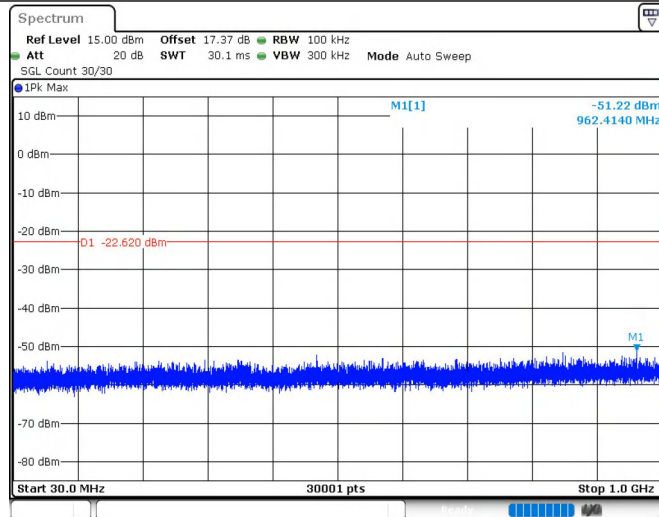
11G_Ant1_2462_30~1000
