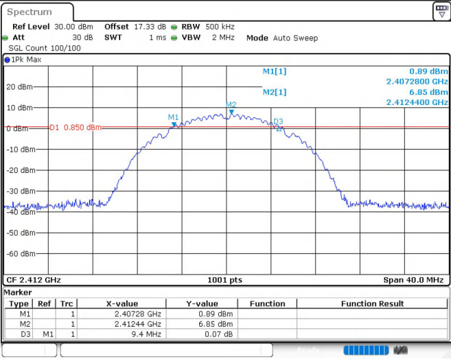
11B_Ant1_2412
