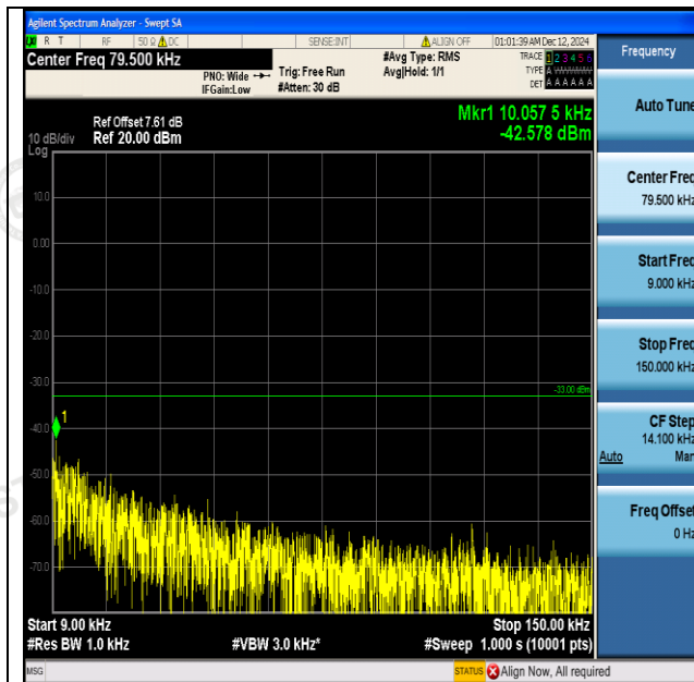
GSM850-190-5-0.009~0.15MHz-PASS
