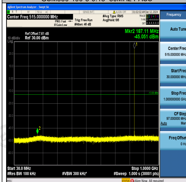
GSM850-190-5-30~1000MHz-PASS
