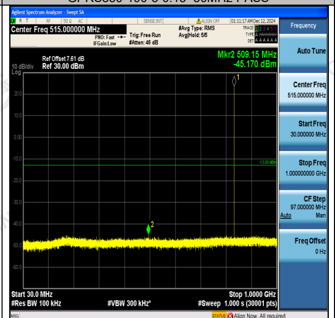
GPRS850-190-5-30~1000MHz-PASS
