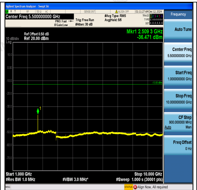
GPRS850-190-5-1000~10000MHz-PASS
